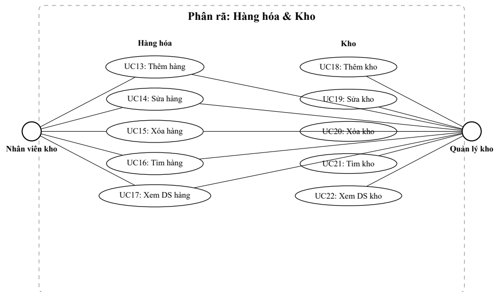
Hình 1: Use case phân rã – Hàng hóa (UC13–17) và Kho (UC18–22)
